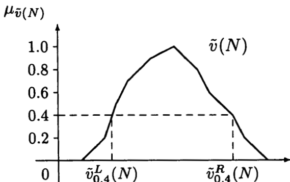
図1 提携 N ファジィ提携値
